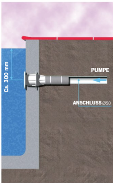
INSTALLATION VON DÜSEN
