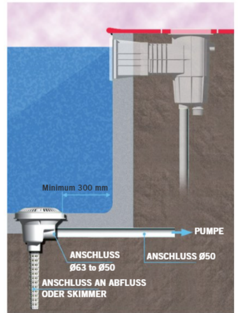
EINBAU DES HAUPTABFLUSSES
