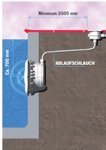
UNTERWASSEREINBAU
