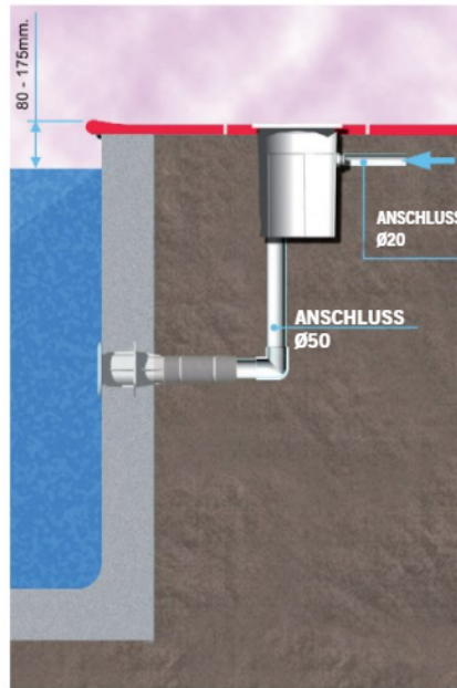
INSTALLATION DES WASSERSTANDSREGLERS
